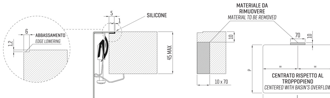
FILOTOP - DETTAGLIO DI FISSAGGIO FLUSH MOUNT - FASTENING DETAIL
