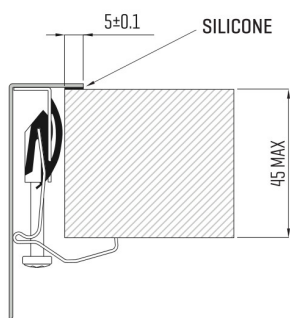
SOPRATOP - DETTAGLIO DI FISSAGGIO TOP MOUNT - FASTENING DETAIL
