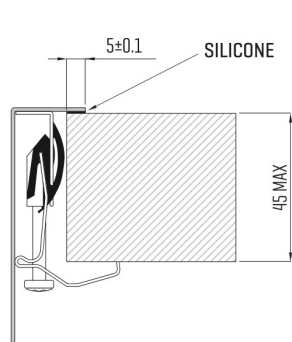
SOPRATOP - DETTAGLIO DI FISSAGGIO TOP MOUNT - FASTENING DETAIL
