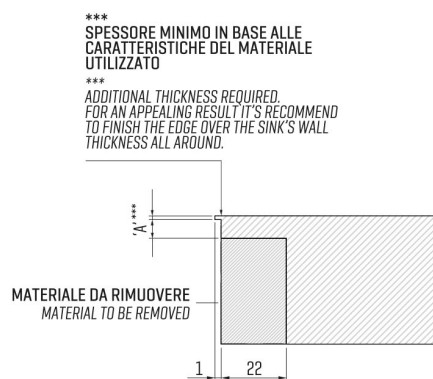
DETTAGLIO ALLOGGIO DEL SUPPORTO SUPPORT HOUSING DETAIL
