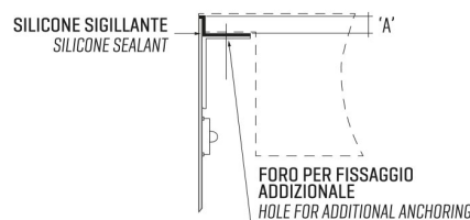
DETTAGLIO DI FISSAGGIO FASTENING DETAIL
