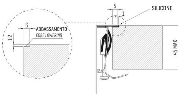
FILOTOP - DETTAGLIO DI FISSAGGIO FLUSH MOUNT - FASTENING DETAIL
